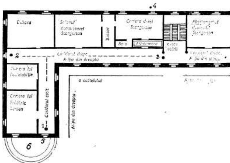
PLANUL PRIMULUI ETAJ AL CASTELULUI (aripa dreaptă).
